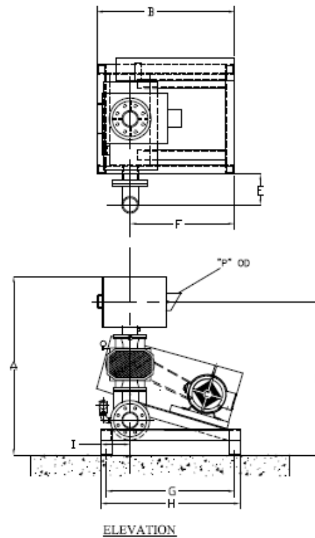
ELEVATION
